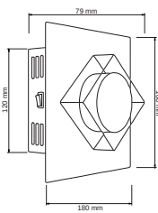
NUEVO TLLED-501/7W/CR FONTANA I
