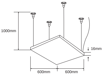
PAN-LED/45W NIZHNI II 30/F: BLANCO CÁLIDO 40/F: BLANCO FRÍO
