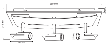
LVC-2003/S CAMENARO I
