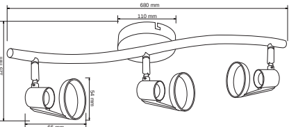
LVR-7203/S BRUSELAS I
