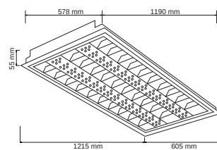
LTL-3280 OFICIOI 41: BLANCO FRÍO 65: LUZ DE DÍA Powered by PHILIPS
