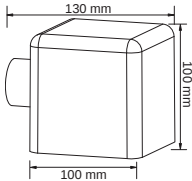
HLED-160 CROSS B: BLANCO S: SATINADO
