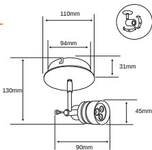
NUEVO LVCLED-01/4W/30AL BAOTOU
