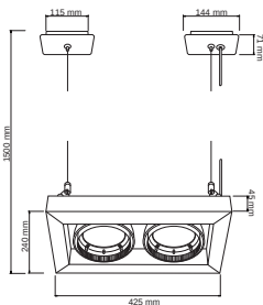
CTL-1112/B LIBIA I
