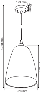
CTL-8083 LUBECK AM: ÁMBAR RO: ROJO OP: OPALINO
