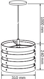
CTL-8170/M LOSANNA I
