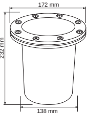
H-625/N CUENCA I
