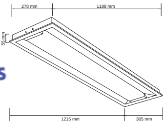
LTL-1540/41 MALMO II
