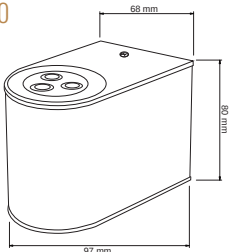
NUEVO HLED-810/6W/40 ABIYÁN
