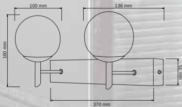
NUEVO TL-4120/CR COMORAS I
