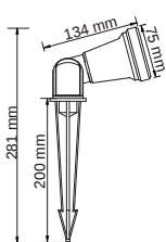
HFV-750/N BILBAO III
