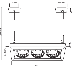
CTL-1113/B LIBIA II
